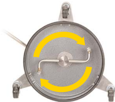
Vista de la parte inferior Brazos rotativos turbo con boquillas duales 1/2"/1.27 cm por encima de la superficie.
